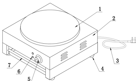
1 : Iron plate 2 : Body 3:Wire 4 : Foot 5 : Thermostat 6 : Light 7 : Debris basin
