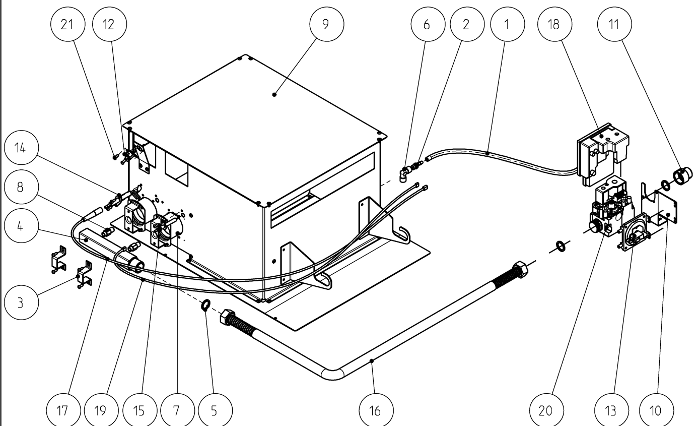
Batteria gas completa Es 10/14/18
