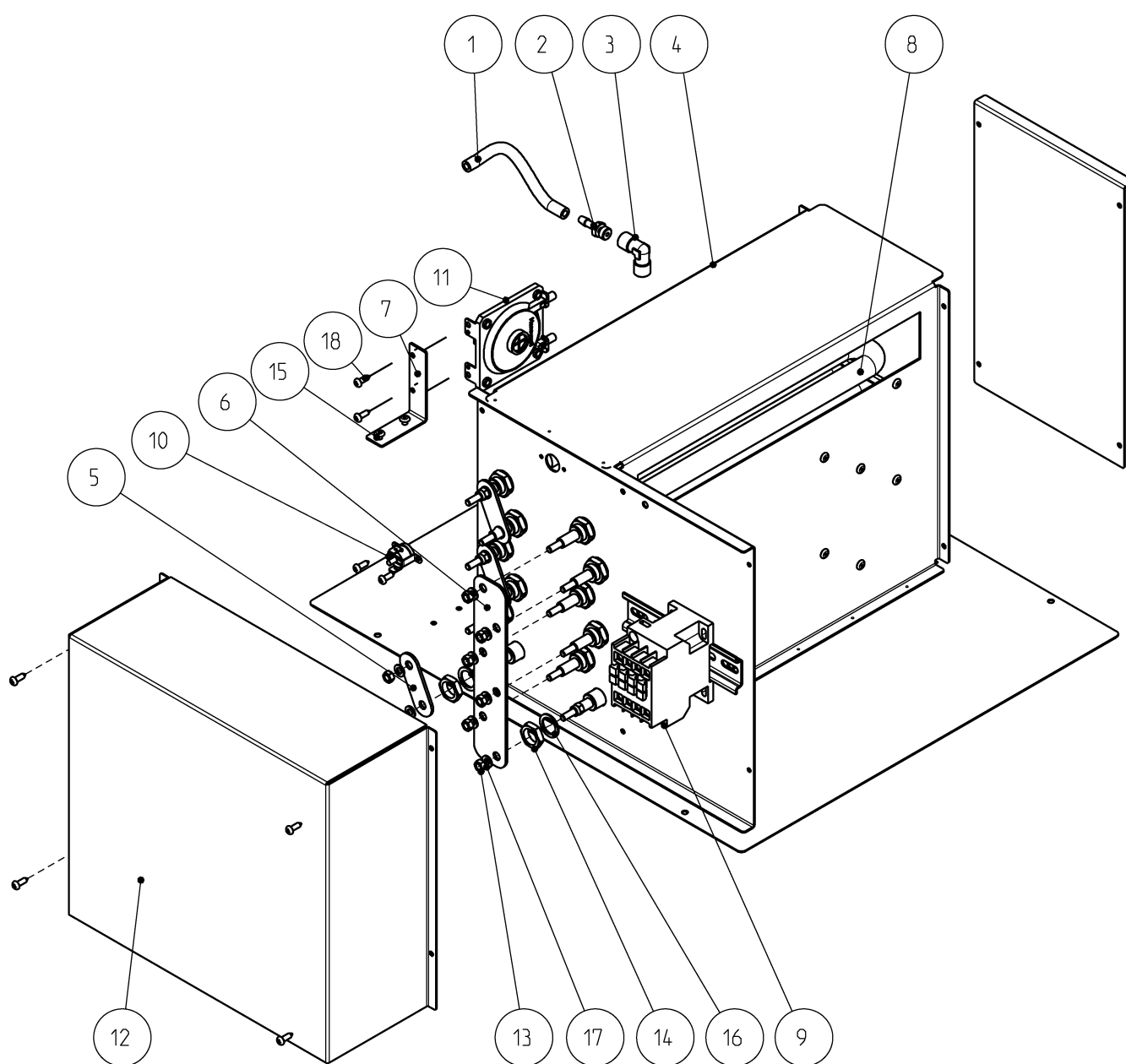
Batteria elettrica completa Es 10/14
