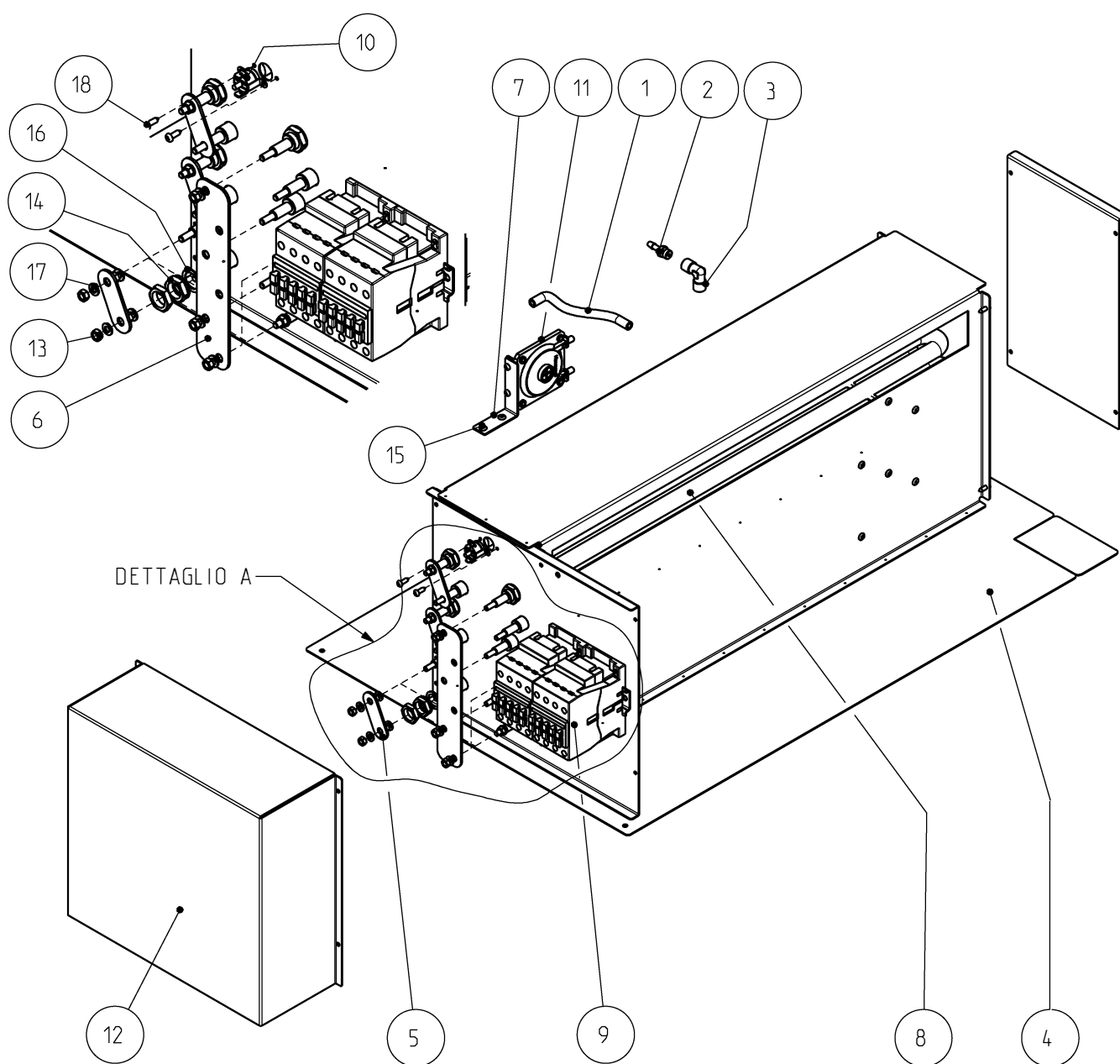
Batteria elettrica completa Es 18/23
