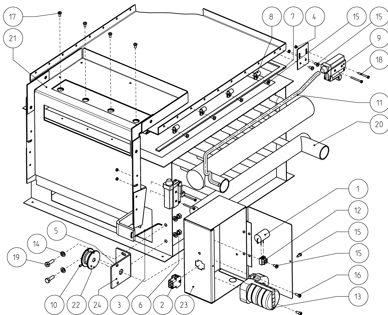
Batteria vapore ES 10/14/18
