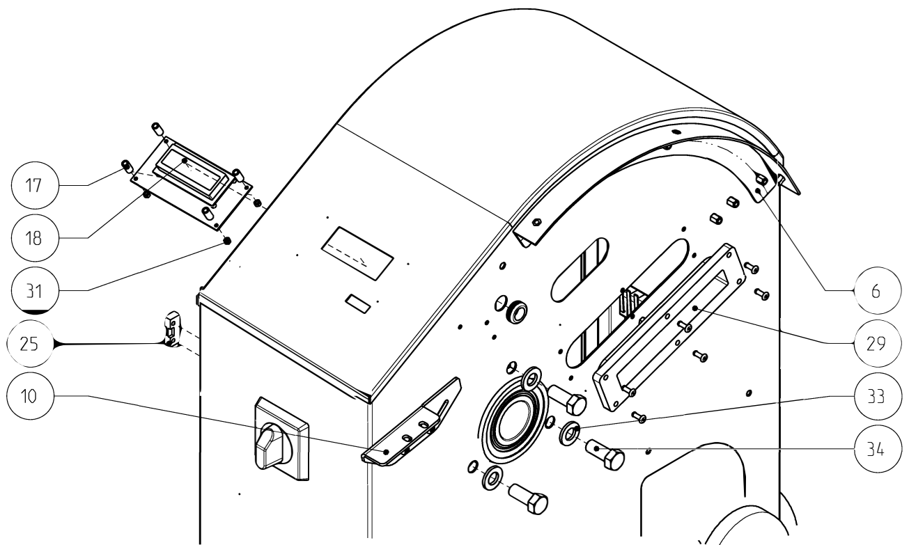
Assieme spalla sinistra mangano
