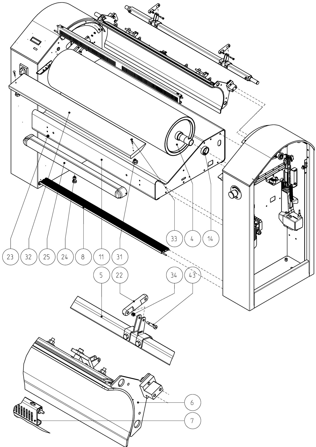
Assieme meccanica mangano
