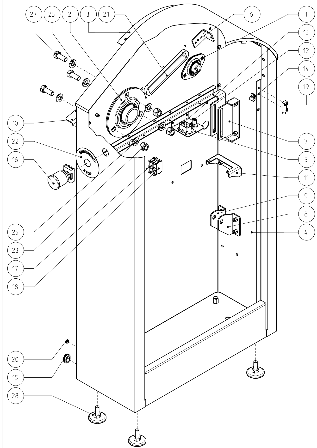
Assieme spalla destra mangano
