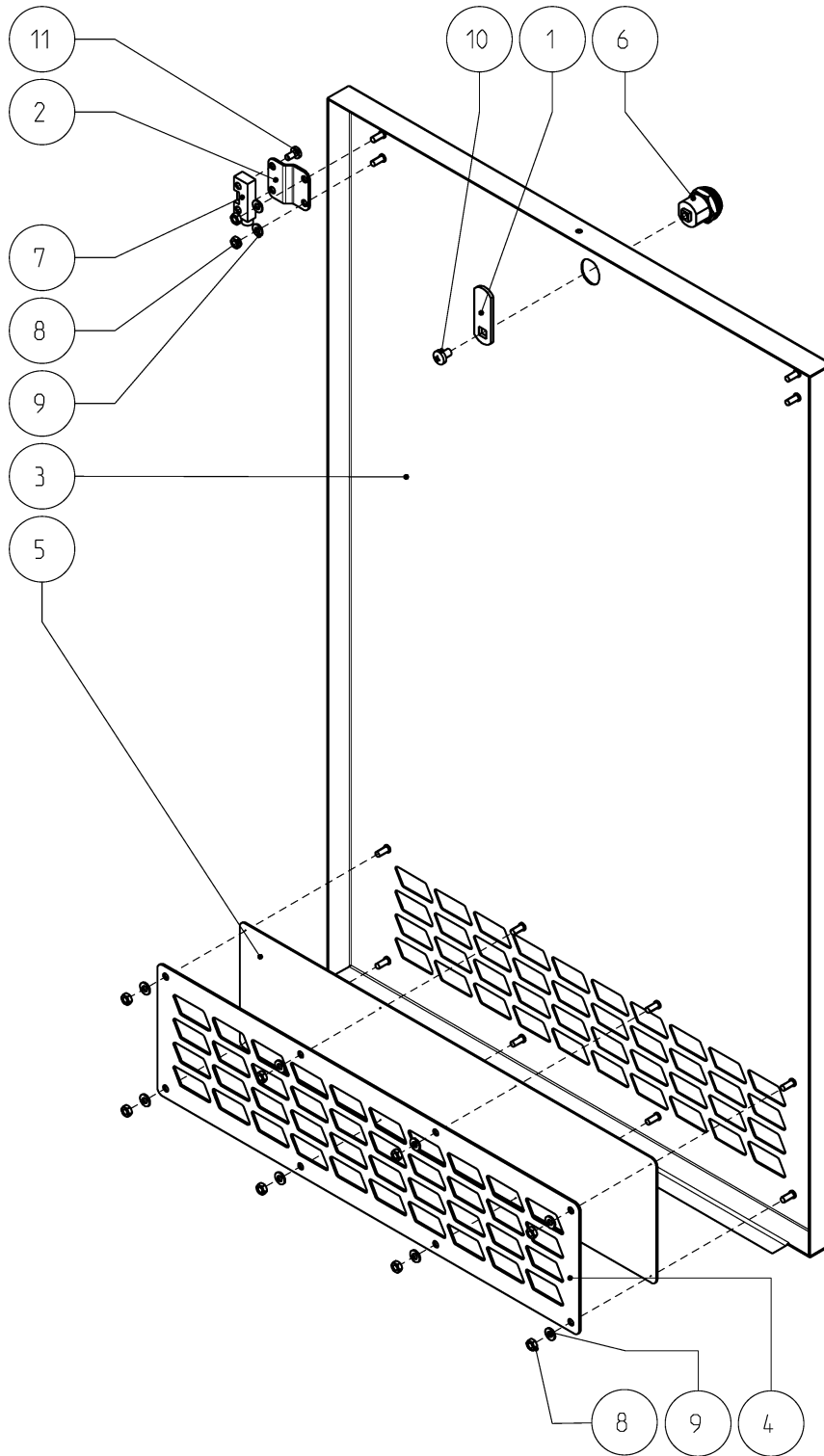
Assieme fianco mangani
