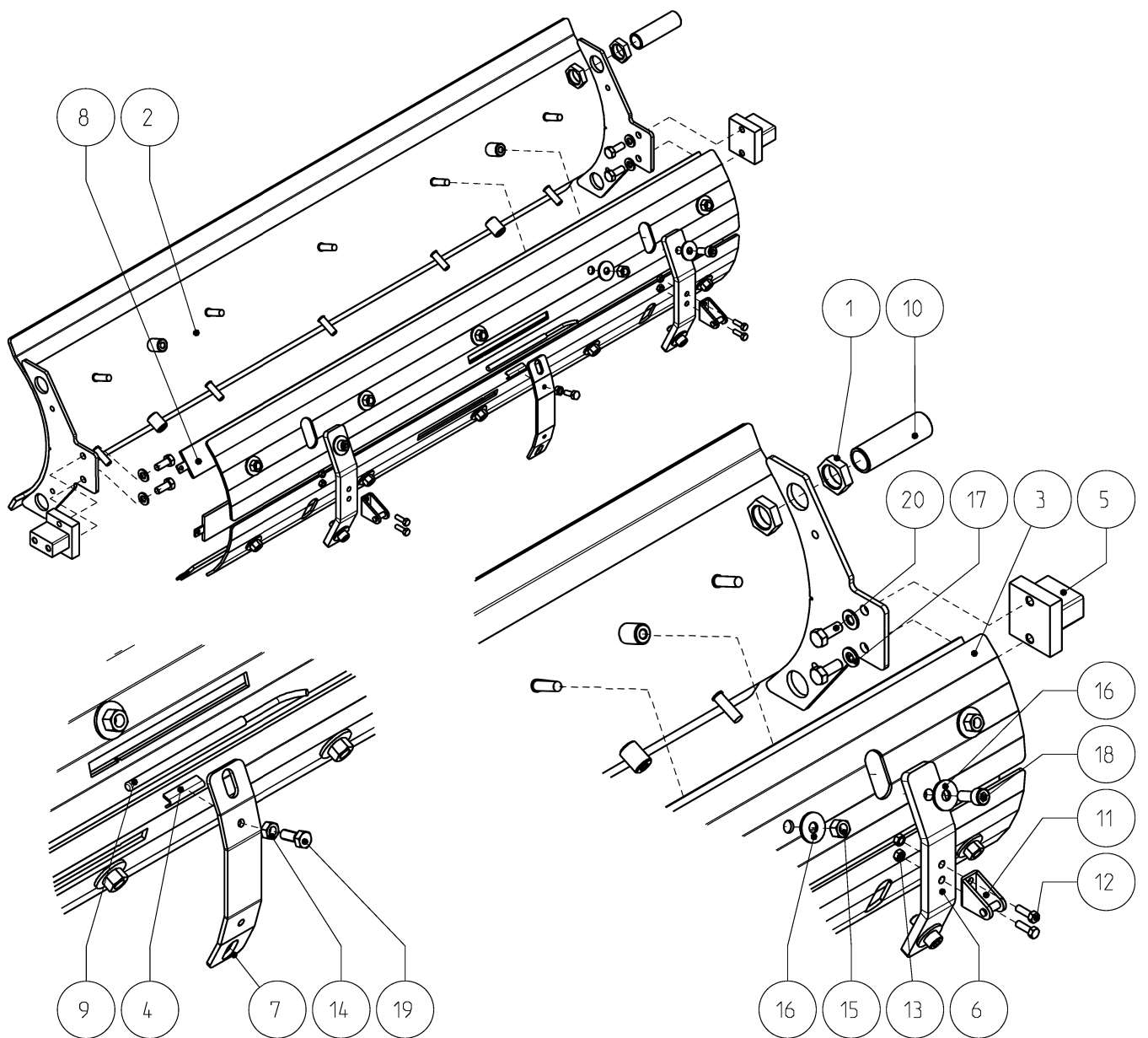
Assieme conca di stiratura mangano
