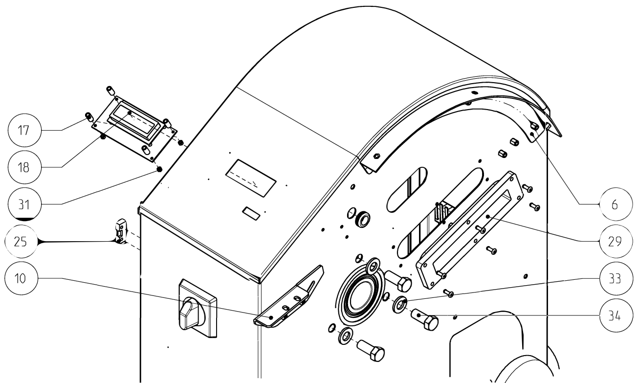
Assieme spalla sinistra mangano FI 1000-1250-1500/25
